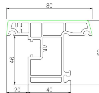
外开扇 B2 SPC60B2-04
