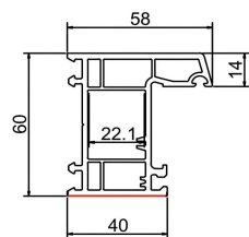
平开框A (小面) SPC60-01A 米重: 1.08Kg/m
