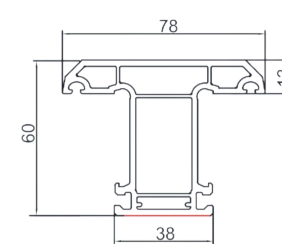
60K外开中挺 SPKB6031B
