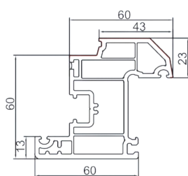
60K内开窗扇 SPKB6020B
