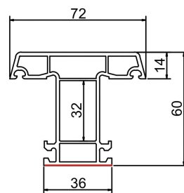
中挺 (小面) SPT60-06 米重: 0.965Kg/m
