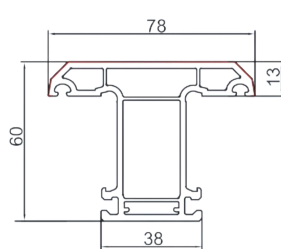
60K内开中挺 SPKB6030B
