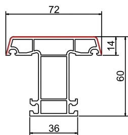
中挺 (大面) SPT60-06 米重: 0.965Kg/m
