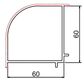
拐角 SPC60-08 米重: 0.72Kg/m
