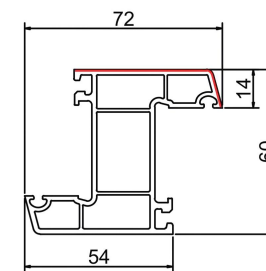
Z型中挺 SPC60Z-20 米重: 1.13Kg/m
