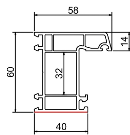
平开框 (小面) SPC60-01 米重: 0.935Kg/m
