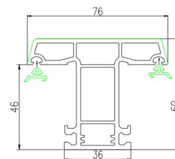
中挺 A2 SPC60A2-03 米重: 1.09kg/m
