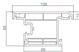
60K外开门扇 SPKB6023 米重: 2.175Kg/m
