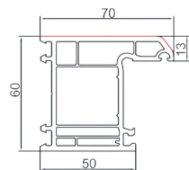
60K内开门框 SPKB6011 米重: 1.53Kg/m
