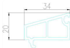
60 单玻压条 PC60DY
