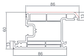
60K内开门扇 SPKB6021 米重: 2.175Kg/m
