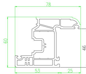
60H 内开扇 SPC60-02H
