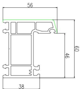
平开框 B2 SPC60B2-01
