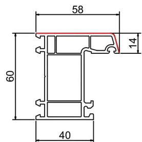
平开框A (大面) SPC60-01 米重: 0.935Kg/m
