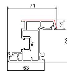
内开扇ASPC60-07A 米重: 1.168Kg/m
