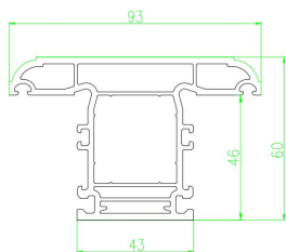
60H 中挺 SPC60-03H
