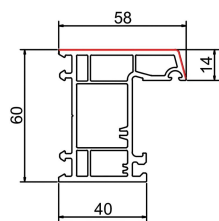
平开框A (大面) SPC60-01A 米重: 1.08Kg/m
