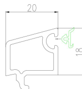
60 双玻压条 PC60SY
