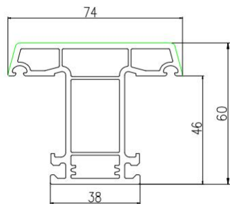
中挺 B2 SPT60B2-02
