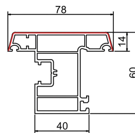
外开扇 SPC60-04 米重: 1.222Kg/m
