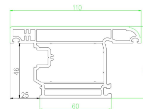
60H 外开扇 SPM60-06H
