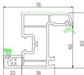
内开扇 A2 SPC60A2-02 米重: 1.15kg/m
