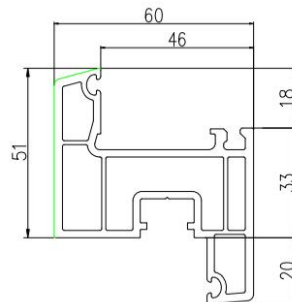
内开扇 B2 SPC60B2-03
