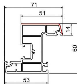
内开扇 SPC60-07 米重: 1.02Kg/m
