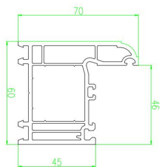
60H 平开框 SPC60-01H
