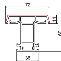
中挺A (大面) SPC60-06A 米重: 1.124Kg/m
