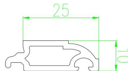
60H 三玻压条 SPCH60-8
