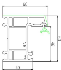
平开框 A2 SPC60A2-01 米重: 1.03kg/m
