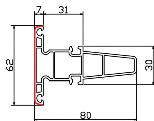
上亮挺 STC80-14 米重: 0.88Kg/m
