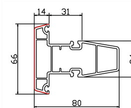
80A上亮中挺 STC80-34 米重: 1.09Kg/m
