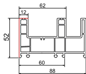
推拉框 STC88-01 米重: 1.324/m
