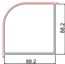
90转角 STC88-13 米重: 1.128Kg/m
