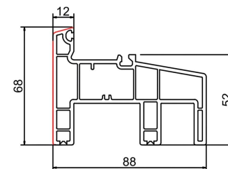
连体框 STC88-16 米重: 1.45Kg/m
