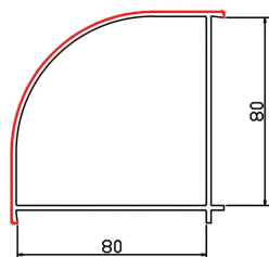
拐角 STC80-13 米重: 0.90Kg/m
