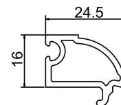
单玻压条 STC88-11 米重: 0.193Kg/m
