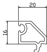
80A单玻压条 STC80-36 米重: 0.187Kg/m 玻璃 5mm
