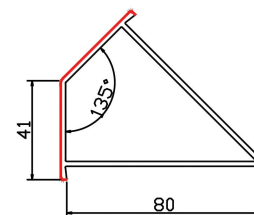
135拐角 STC80-23 米重: 0.79Kg/m
