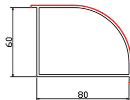
60/80拐角 STC80-26 米重: 0.77Kg/m
