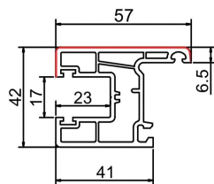
推拉扇 (B) STC88-06 米重: 0.813Kg/m
