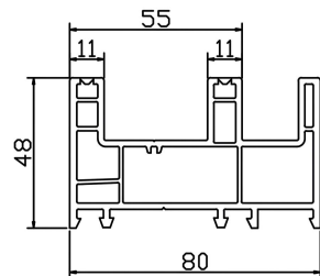
推拉框 DSTC80-04 米重: 1.00Kg/m
