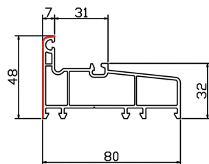
上亮框 BSTC80-11 米重: 0.84Kg/m
