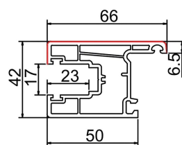
推拉扇 (A) STC88-02 米重: 0.926Kg/m
