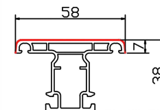
扇挺 STC80-12 米重: 0.625Kg/m
