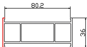
拼管 STC80-24 米重: 0.735Kg/m
