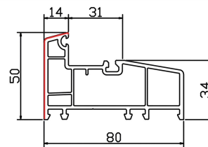
80A上亮框 STC80-33 米重: 1.02Kg/m
