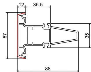
固定中挺 STC88-05 米重: 1.062Kg/m
