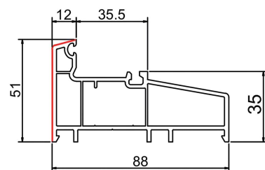
A固定框 STC88-04A 米重: 1.15Kg/m
