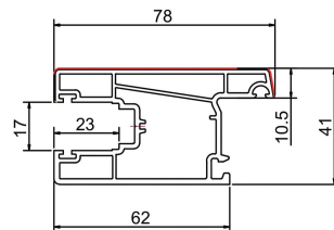
推拉门扇 STC60-02 米重: 1.00Kg/m
