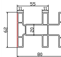
王字框 STC80-15 米重: 1.30Kg/m
