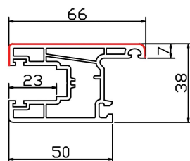
推拉扇 ASTC80-06 米重: 0.78Kg/m
