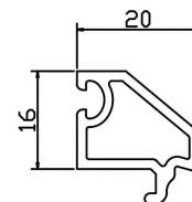
80A单玻压条 STC80-36 米重: 0.187Kg/m 玻璃 5mm
