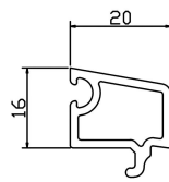
推拉单玻 STC80-20 米重: 0.172Kg/m 玻璃 5mm
