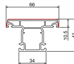
60推拉门扇 STC60-04 米重: 0.726Kg/m
