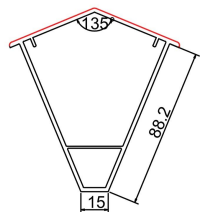
135转角 STC88-12 米重: 1.128Kg/m
