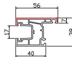
推拉扇 BSTC80-07 米重: 0.70Kg/m
