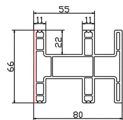
80A王字框 STC80-35 米重: 1.56Kg/m
