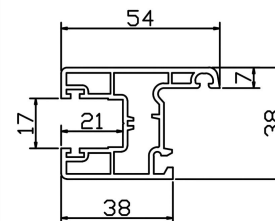
推拉扇 CSTC80-08 米重: 0.65Kg/m
