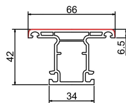
推拉扇挺 STC88-07 米重: 0.742Kg/m
