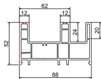
A推拉框 STC88-01A 米重: 1.56Kg/m
