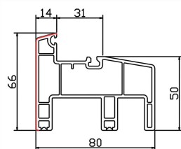
80A连体框 STC80-32 米重: 1.33Kg/m
