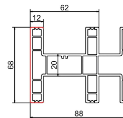
王字框 STC88-03 米重: 1.639Kg/m
