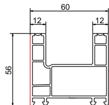
二轨框 STC80-01 米重: 1.00Kg/m
