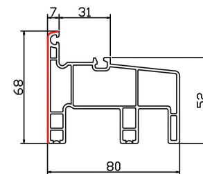
连体框 STC80-09 米重: 1.20Kg/m
