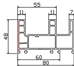
推拉框A2 STC80-02 米重: 1.10Kg/m
