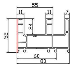
推拉框A1 STC80-01 米重: 1.33Kg/m
