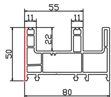
80A推拉框 STC80-31 米重: 1.25Kg/m
