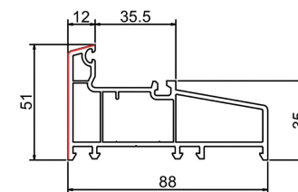
固定框 STC88-04 米重: 0.993Kg/m
