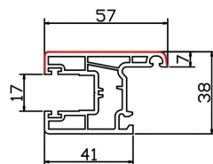
57扇 STC80-05 米重: 0.81Kg/m
