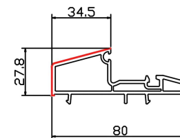
一体盖帽 STC80-18 米重: 0.52Kg/m
