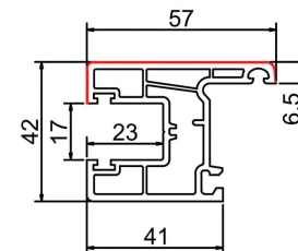
A推拉扇 (B) STC88-06A 米重: 0.98Kg/m
