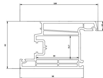
65K 内开门扇 SPM65K-01-06
