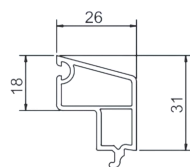
65框挺双玻C SPC65-12-12 米重: 0.294Kg/m 玻璃 5+9+5
