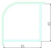
65-90° 转角
