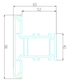
65A2 中挺 SPC65A2-01-03 米重: 1.51kg/m
