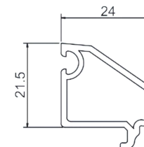
65G双玻 SPC65G-01-5 米重: 0.22Kg/m
