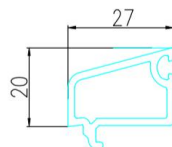
65 扇双玻压条 SPC65K-02-04
