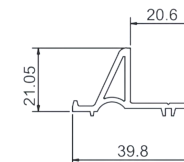
垫桥 SPC65-11-06 米重: 0.24Kg/m
