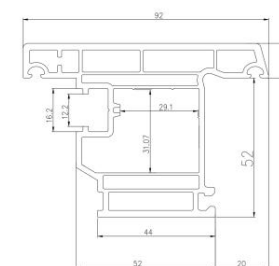
65K 外开扇 SPC65K-01-03 米重: 1.45kg/m
