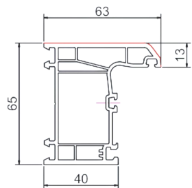
65G平开框 SPC65G-01-01 米重: 1.10Kg/m
