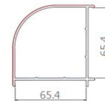
转角 SPC65-09 米重: 0.883kg/m
