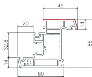
内开扇 SPC65-02-03 米重: 1.4Kg/m
