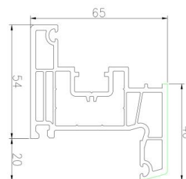
65K 内开扇 SPC65K-01-02 米重: 1.225kg/m
