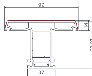
平开中挺 SPC65-03-04 米重: 1.349Kg/m
