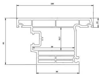
65K 外开门扇 SPM65K-01-05
