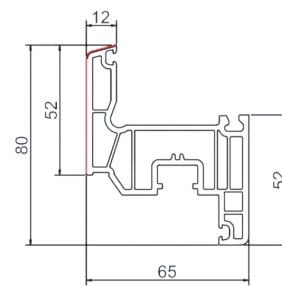
65内开扇 SPC65A-02-7 米重: 1.46Kg/m
