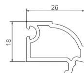
双玻压条 SPC65-04-09 米重: 0.219Kg/m 玻璃 5+9+5
