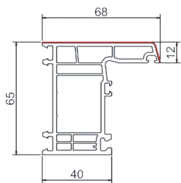
65平开框 SPC65-01-01-A 米重: 1.327Kg/m
