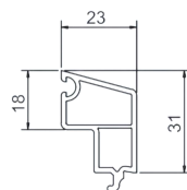
65框挺双玻B SPC65-10-08B 米重: 0.27Kg/m 玻璃 5+12+5
