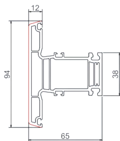
65中挺 SPC65-01-4 米重: 1.527Kg/m
