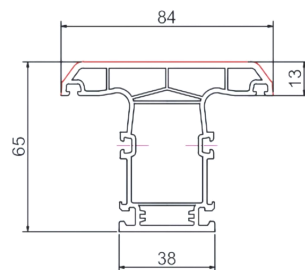
65G SPC65G-01-4 米重: 1.27Kg/m
