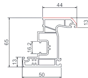
65G内开 SPC65G-02 米重: 1.14Kg/m
