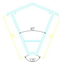
65-135° 转角
