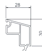
65框挺双玻A SPC65-07-07 米重: 0.29Kg/m 玻璃 4+9+4
