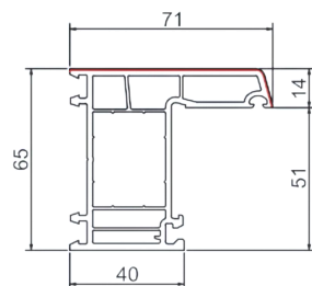
平开框 SPC65-01-01 米重: 1.175Kg/m
