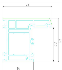
65A2 平开框 SPC65A2-01-01 米重: 1.39kg/m
