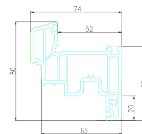
65A2 内开扇 SPC65A2-01-02 米重: 1.54kg/m
