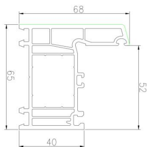
65K 平开框 SPC65K-01-01 米重: 1.18kg/m
